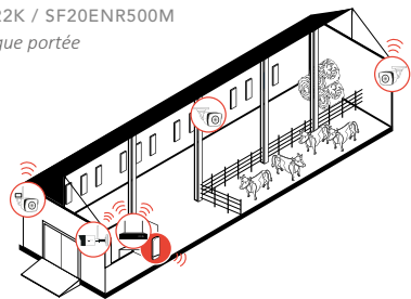
Option Op. Caméras longue portée Réf. : SF20ANTEX Transmission longue portée pour les caméras 1km à vue
